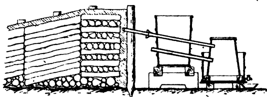
Fig. 20. — Condenseur pour l'acide pyroligneux.
